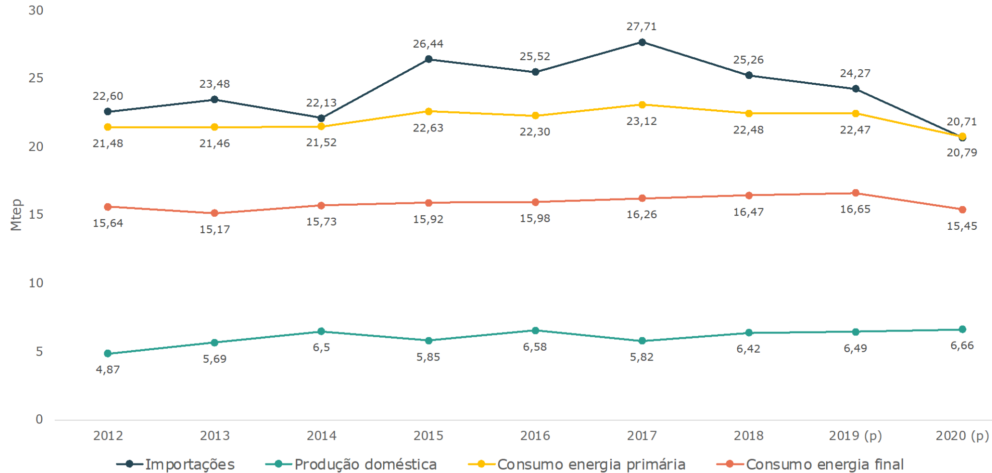
Balço energético - Importações, produção doméstica e consumos de energia primária e de energia final, em Portugal | 2012-2020
