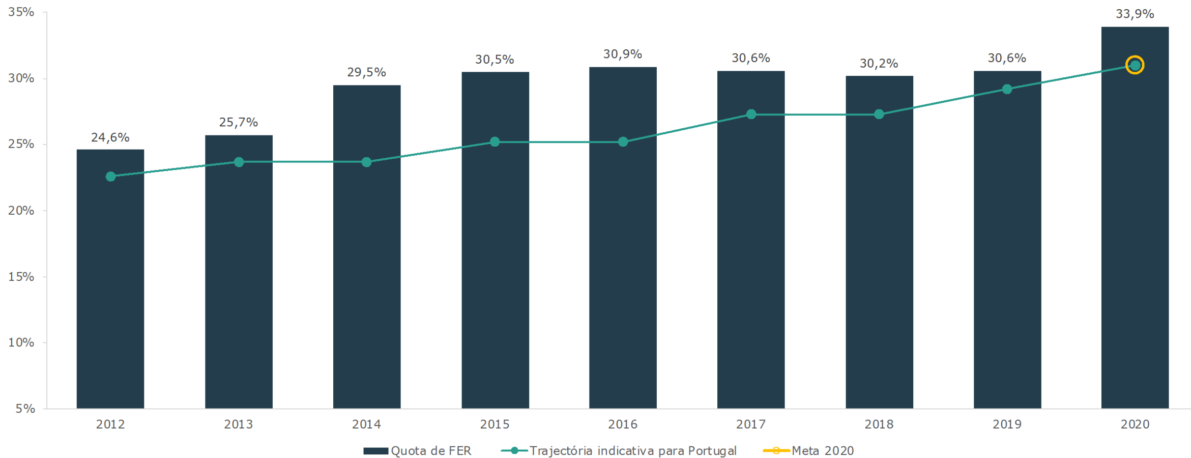
Peso das fontes de energia renovável (FER) no consumo final bruto de energia, em Portugal | 2012-2020
