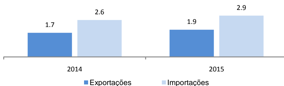
Figura 1 – Peso da pesca, preparações, conservas e outros produtos do mar nas Exportações e nas importações totais portuguesas (%) - 1º semestre de 2014 e 2015 -
